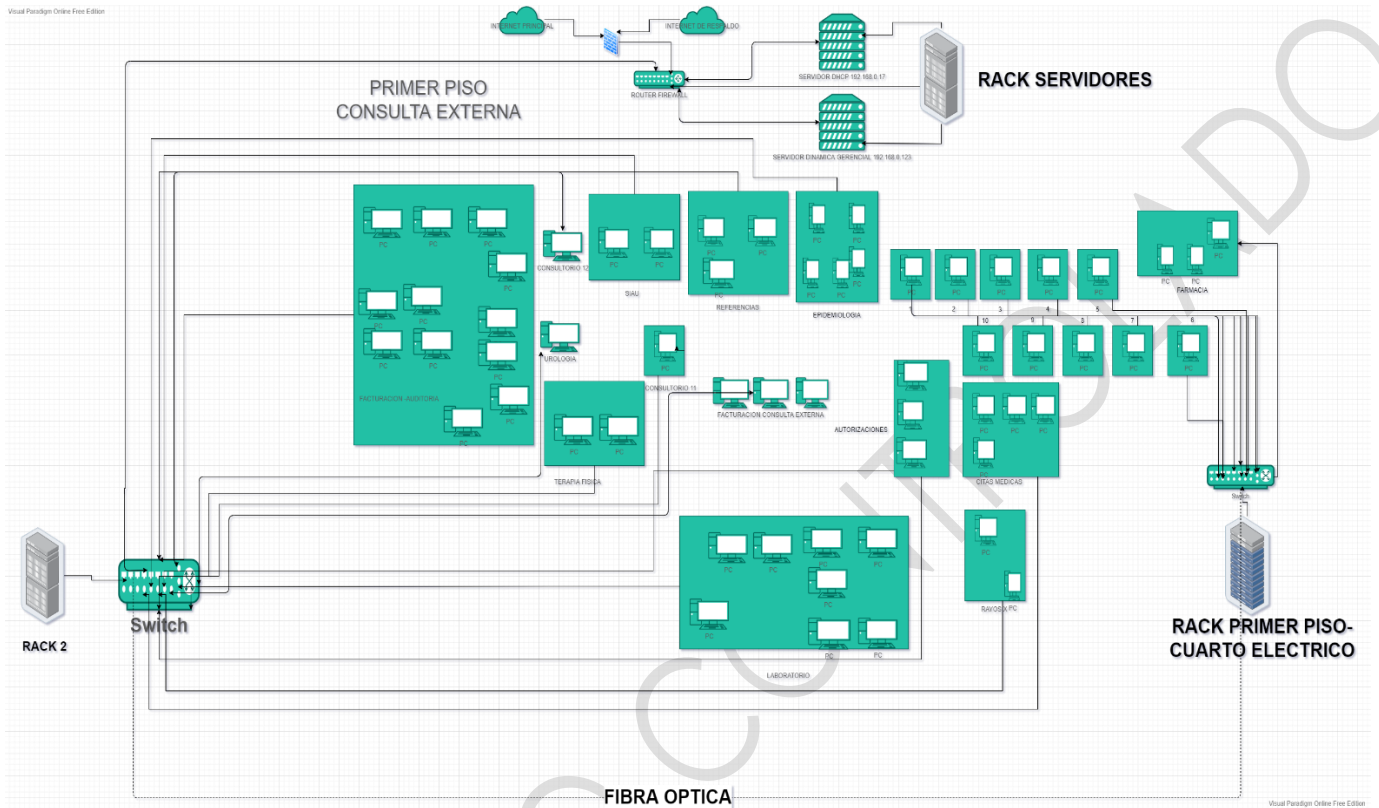
Ilustración 3–Esquema físico de Red de UCI-Urgencias
